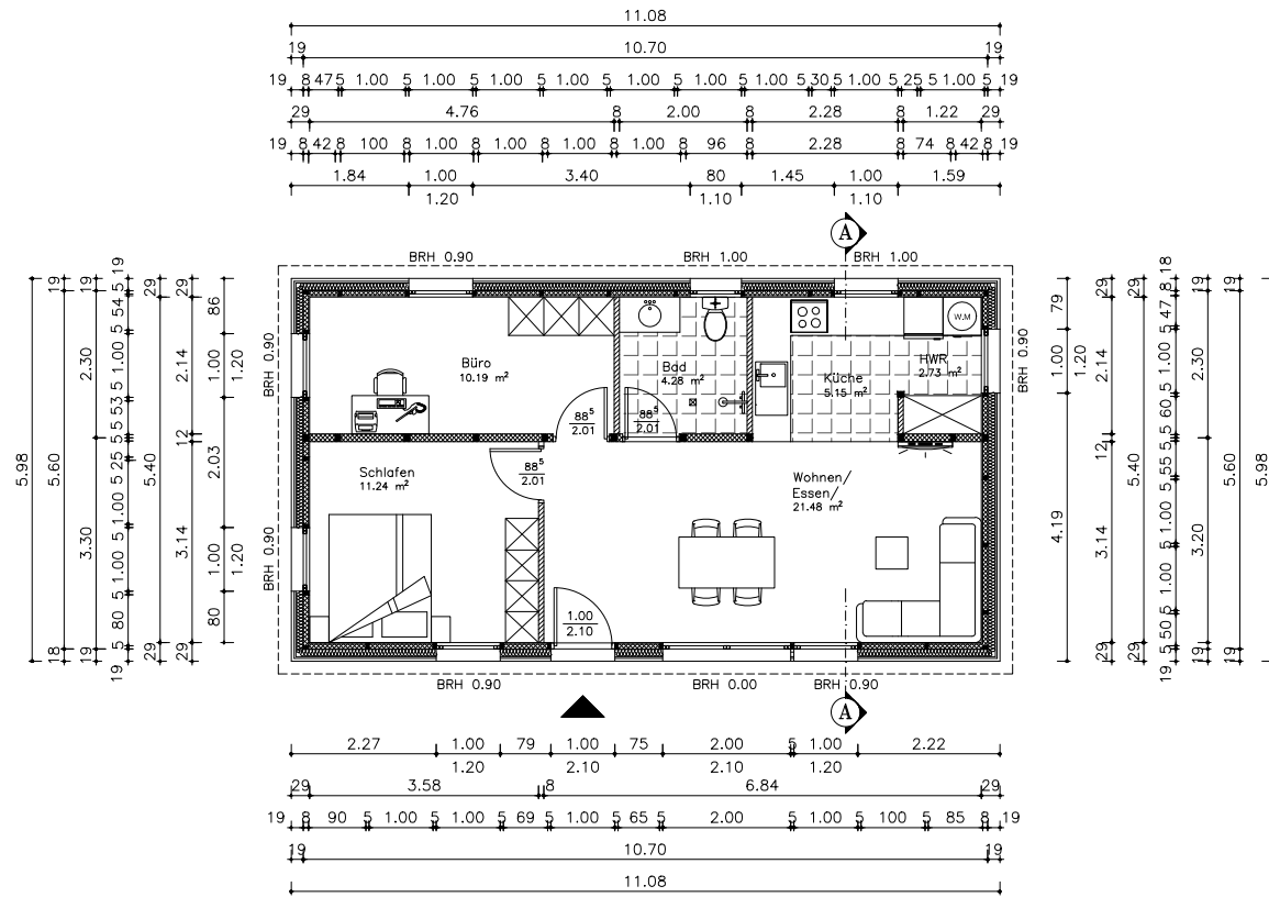
● Grundriss Erdgeschoss
