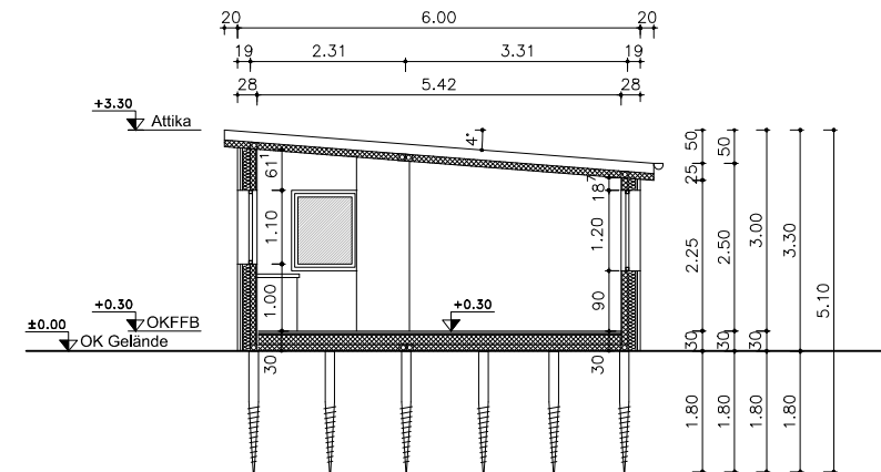
● Ansicht A-A
