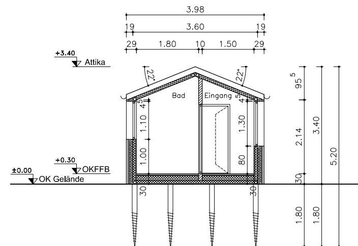
● Ansicht A-A
