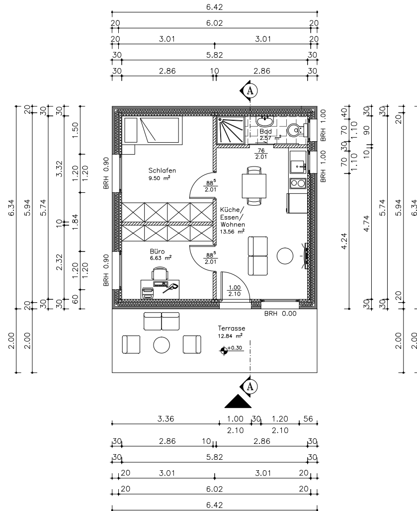
● Grundriss Erdgeschoss
