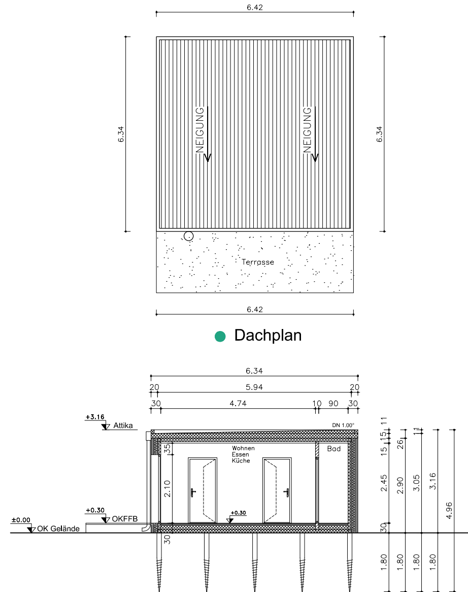
● Ansicht A-A
