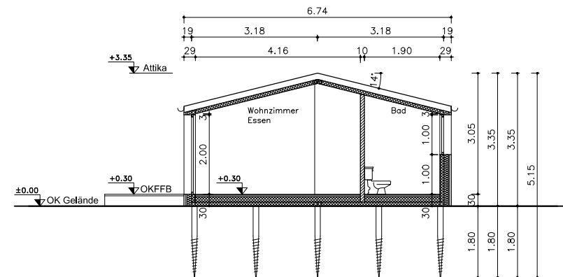
● Ansicht A-A
