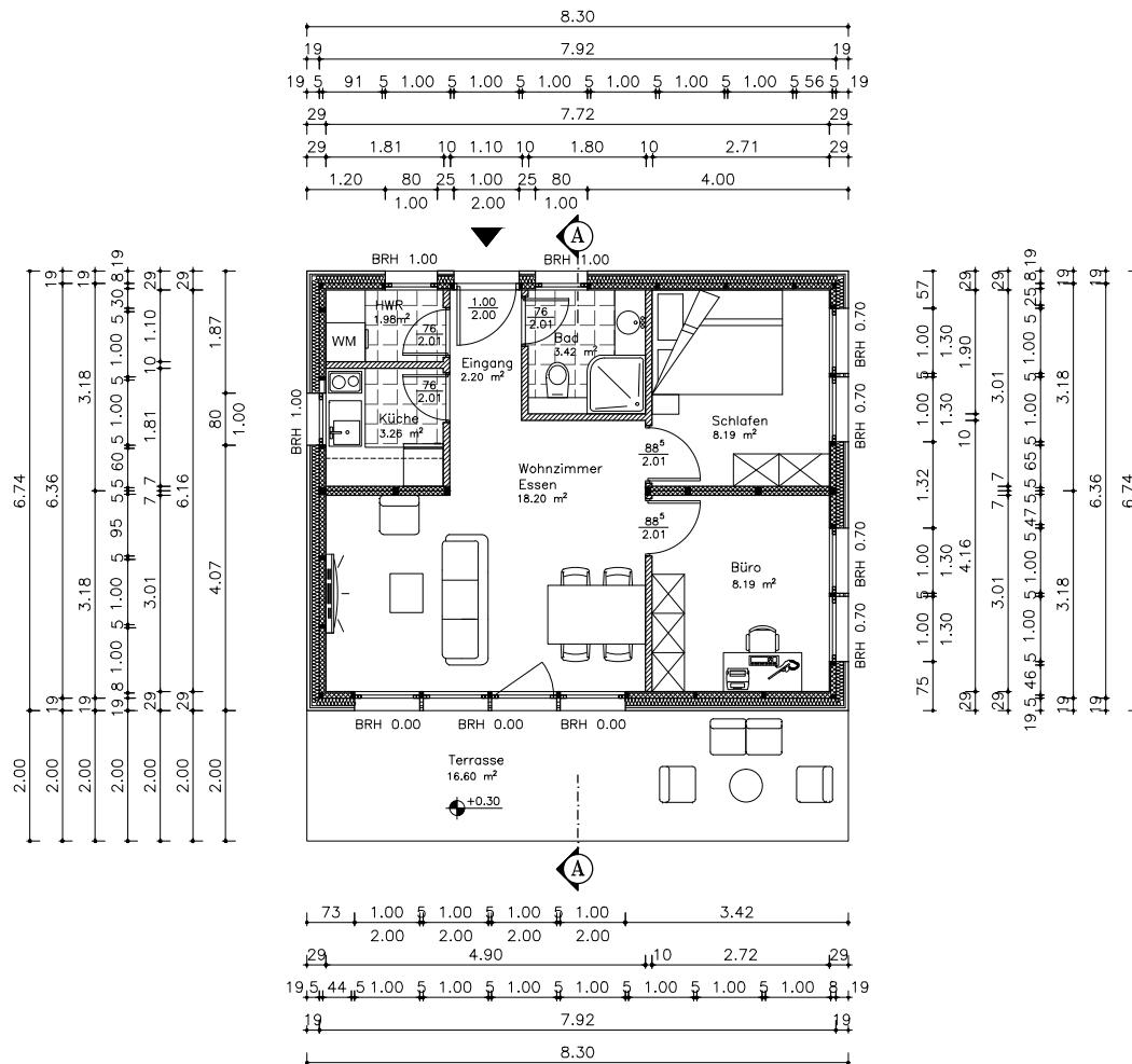
● Grundriss Erdgeschoss
