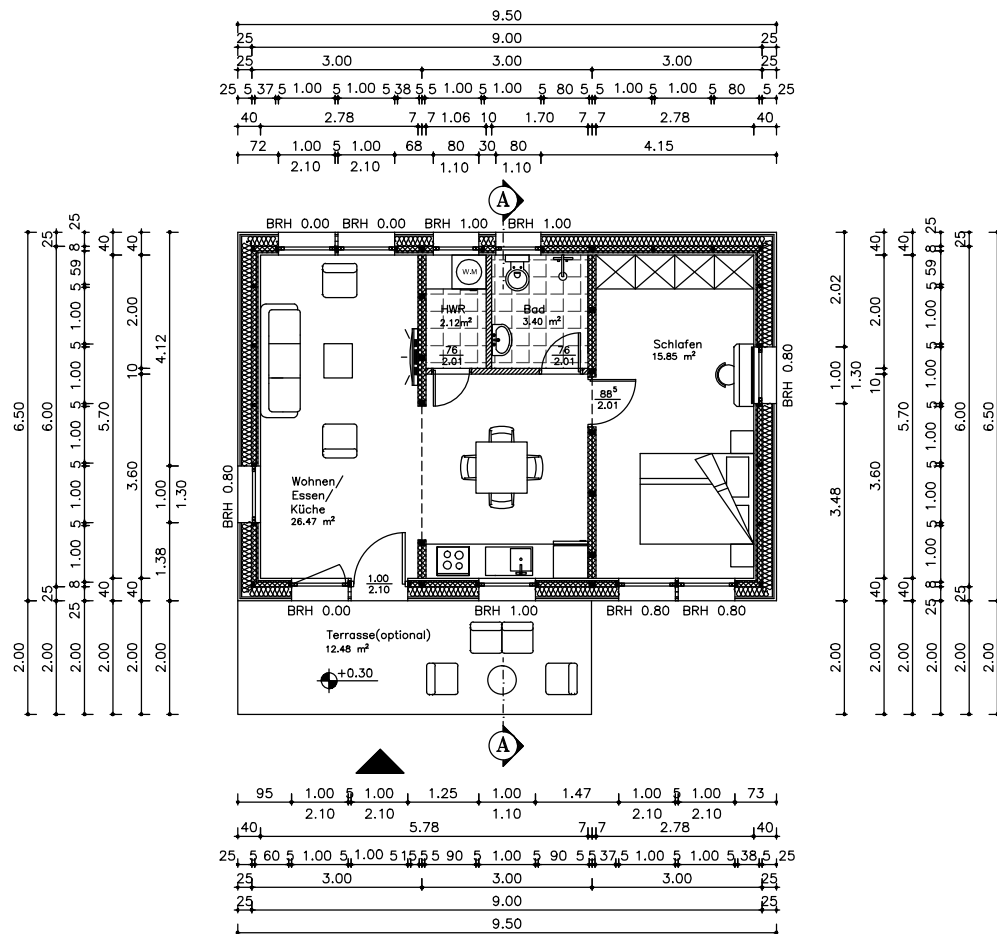
● Grundriss Erdgeschoss
