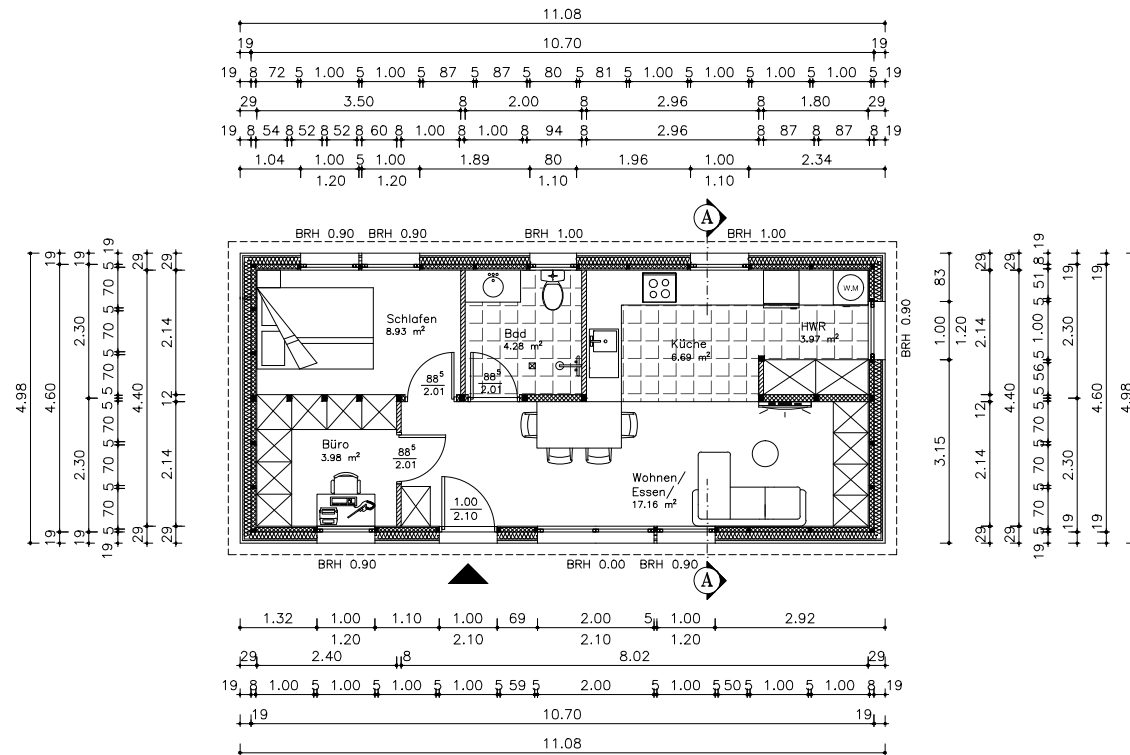
● Grundriss Erdgeschoss
