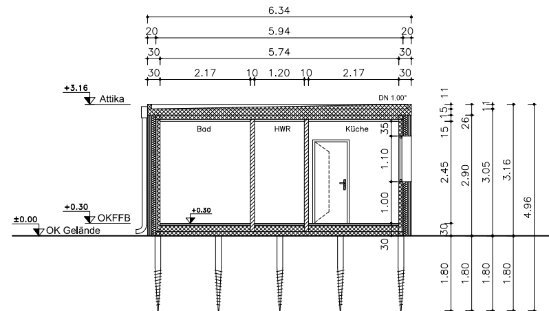
● Ansicht A-A
