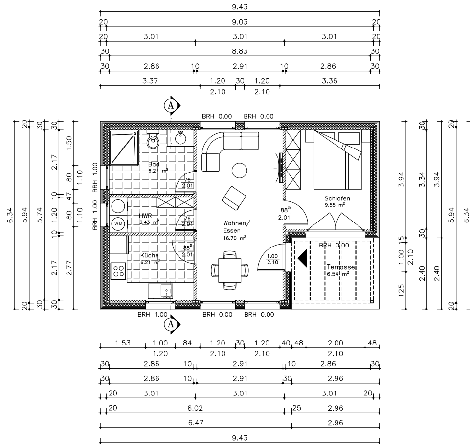
● Grundriss Erdgeschoss
