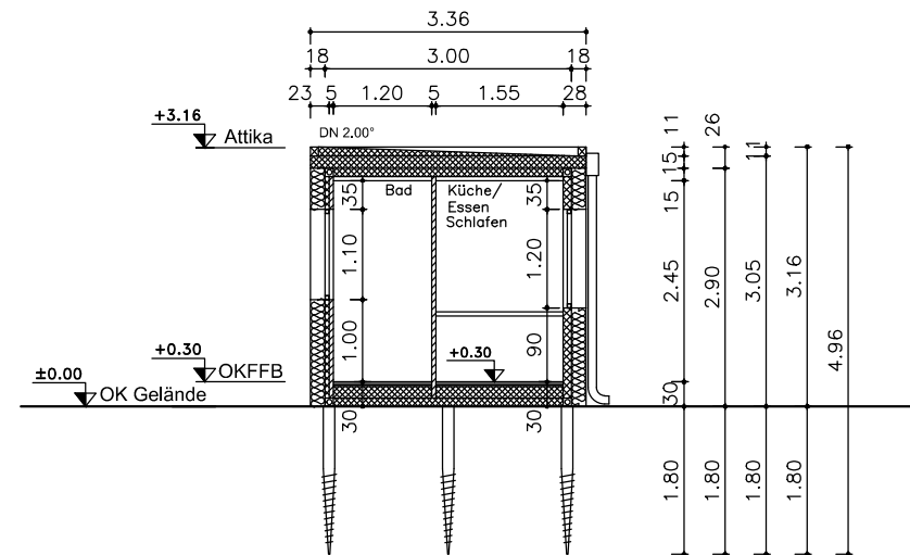
● Ansicht A-A
