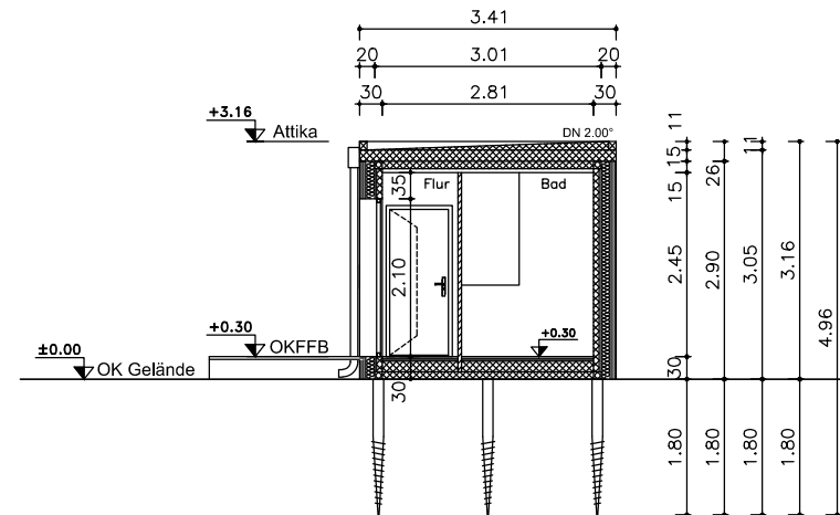
● Ansicht A-A
