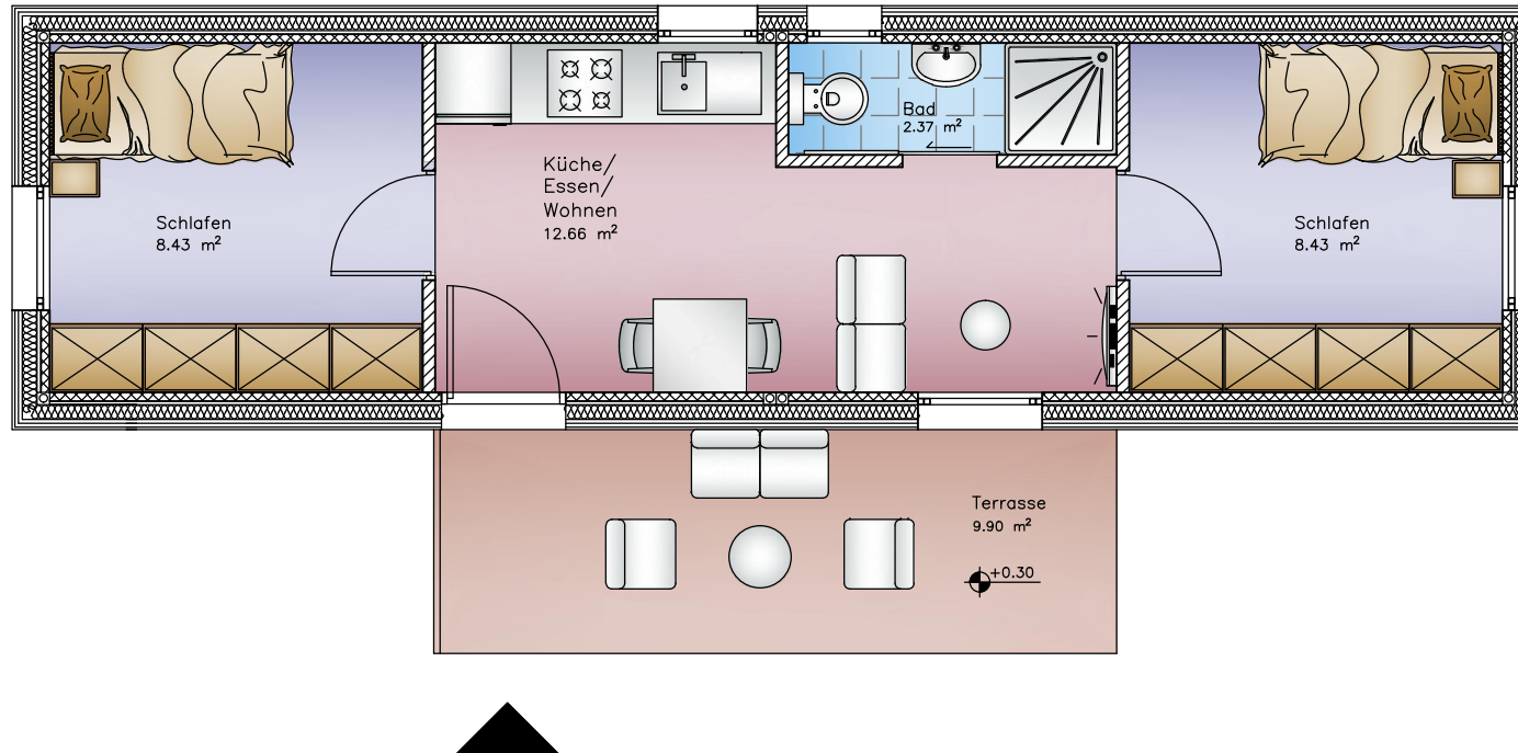
● Grundriss Erdgeschoss
