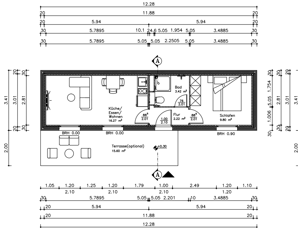
● Grundriss Erdgeschoss
