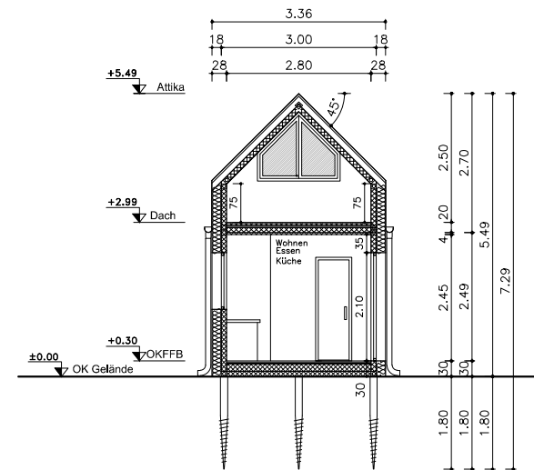
● Ansicht A-A
