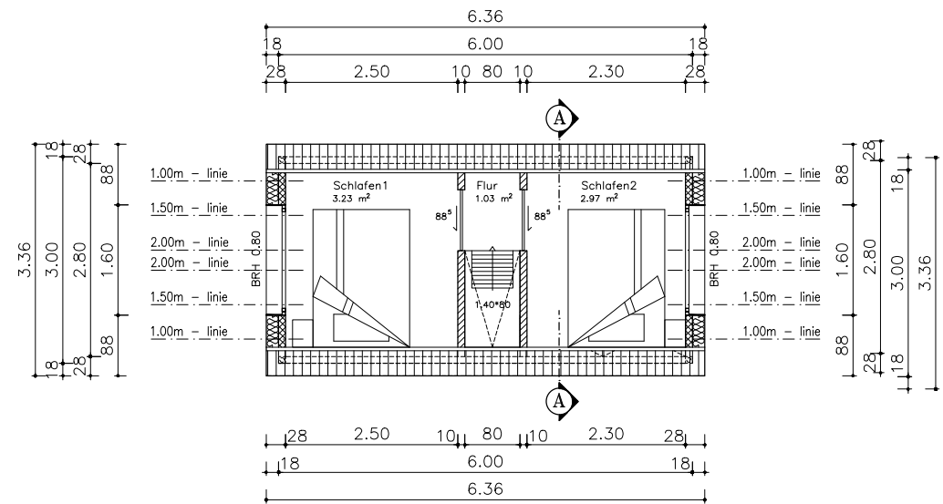
● Grundriss Erdgeschoss
